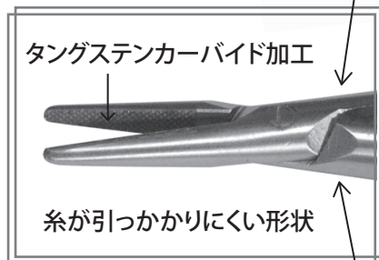
ニードルホルダーカストロビューホ スタンダード TC加工 <縫合糸範囲: 5-0 ~ 6-0>
